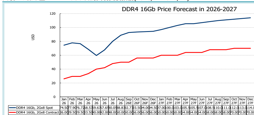
圖表 2：標準型 DDR4 16Gb 合約與現貨價預估(2026/1~2027/12)
